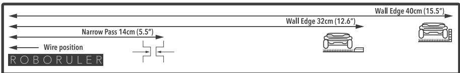
RoboRuler Zum Messen der Entfernung des Begrenzungsdrahtes von der Rasenkante
